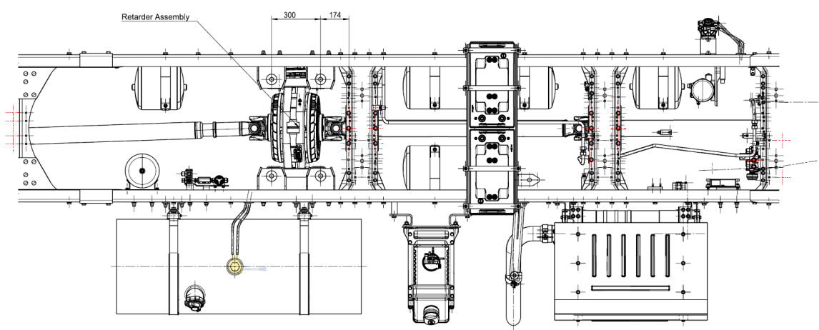
A1 - A1 Disposition of Ad Blue tank
